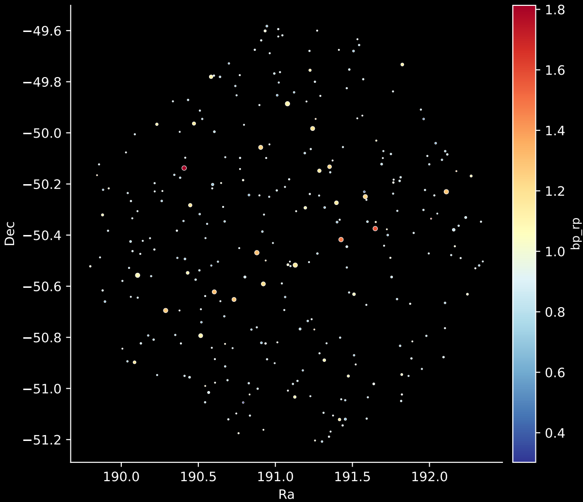
GALAH DR4 Field: [1111] Stars: 298
