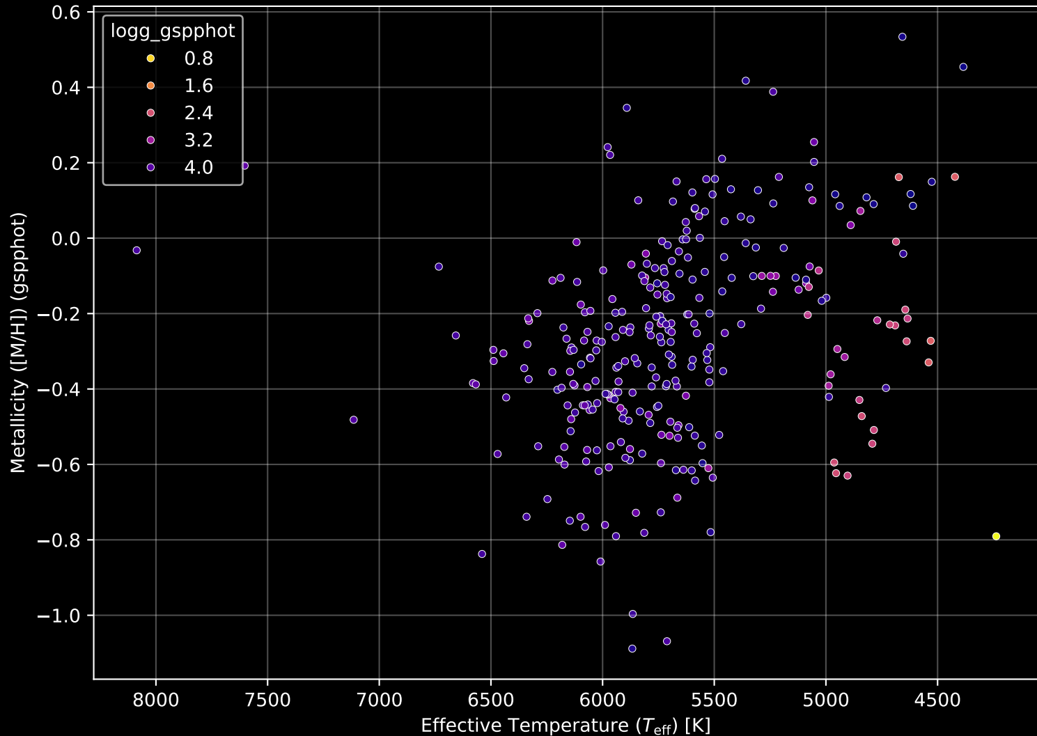
GALAH DR4 Field: [1111] Stellar Population Parameters (n= 298)
