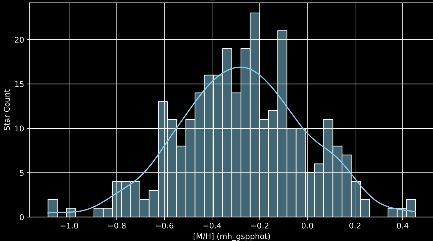
GALAH DR4 Field: [1111] [M/H] (mh_gspphot) (n= 297)
